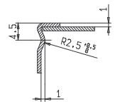
Sezione/Section B-B scala/scale 2:1
