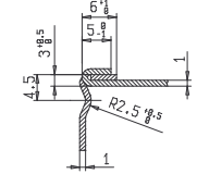
Sezione/Section A-A scala/scale 2:1
